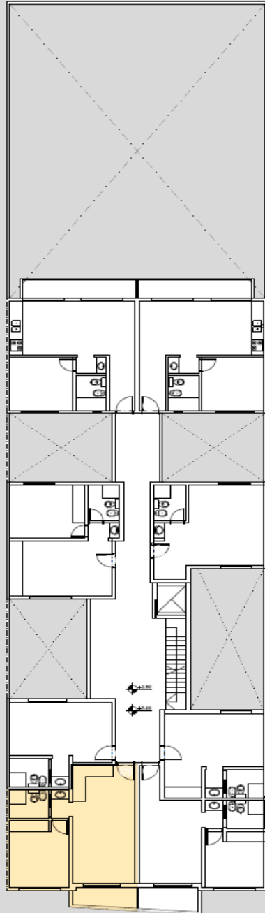
Planta 1° a 3° Piso
